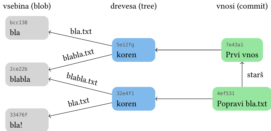
Slika 3: Vsebinsko naslovljiva shramba objektov v Gitu. Naslovi so zgostitve vsebine. Shramba vsebuje dva vnosa. V prvem vnosu smo dodali dve datoteki bla.txt in blabla.txt, v drugem vnosu pa smo spremenili le vsebino datoteke bla.txt.
