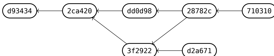
Slika 2: Vnosi v Gitu kot usmerjen graf. Vsak vnos(razen prvega) ima povezavo na vnose iz katerih izhaja. Git hrani zgodovino sprememb v vsebinsko naslovljivi shrambi objektov , ki hrani tri vrste objektov:
