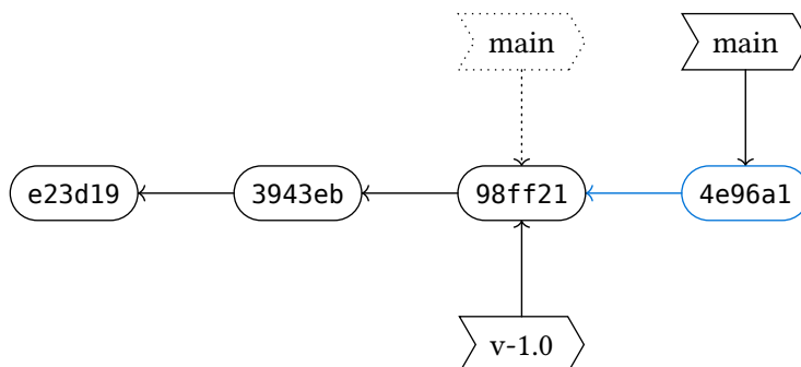
Slika 3: Ko ustvarimo nov vnos, se aktivna veja main premakne naprej, značka v-1.0 pa ostane tam, kjer je bila.
