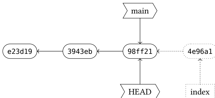
Slika 4: HEAD je referenca na trenutno aktiven vnos/vejo.
