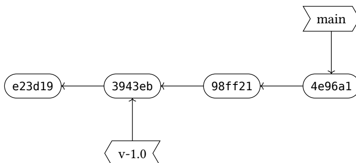
Slika 2: Veja (angl. branch) ali značka(angl. tag) je preprost kazalec na posamezen vnos(angl. commit).
