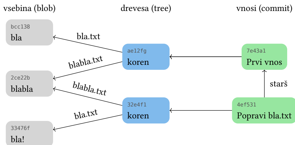
Slika 3: Vsebinsko naslovljiva shramba objektov v Gitu. Naslovi so zgoščene vrednosti vsebine. Shramba vsebuje dva vnosa. V prvem vnosu smo dodali dve datoteki bla.txt in blabla.txt , v drugem vnosu pa smo spremenili le vsebino datoteke bla.txt .
