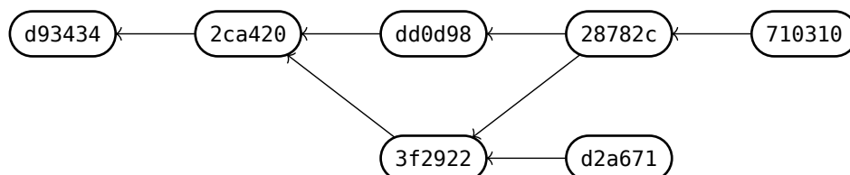
Slika 2: Vnosi v Gitu kot usmerjen graf. Vsak vnos(razen prvega) ima povezavo na vnose iz katerih izhaja. Git hrani zgodovino sprememb v vsebinsko naslovljivi shrambi objektov , ki hrani tri vrste objektov:
